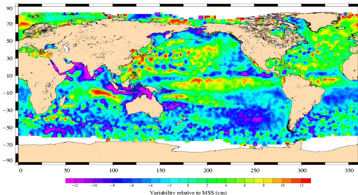
Envisat Cycle 051 04/09/2006 – 09/10/2006
