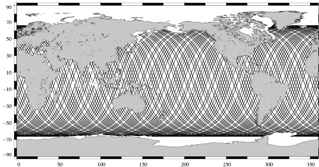
Valid data Jason-1 Cycle 082 (28/03/2004 / 07/04/2004)
