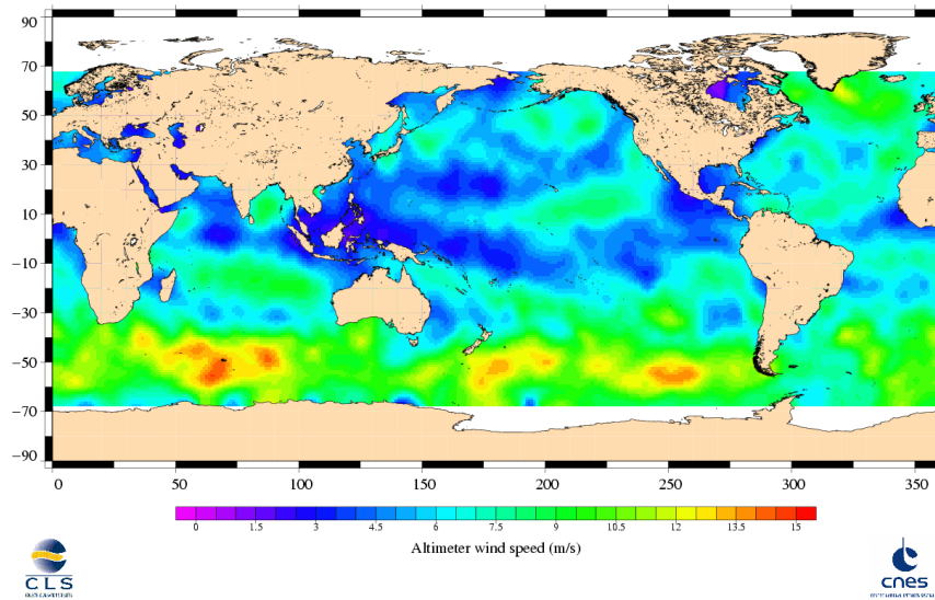
Jason-1 Cycle 197 12/05/2007 - 22/05/2007
