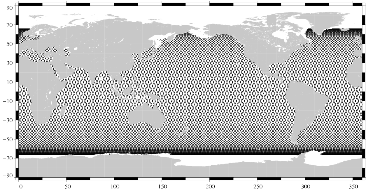
Valid data Jason-1 Cycle 302 (13/03/2010 / 23/03/2010)
