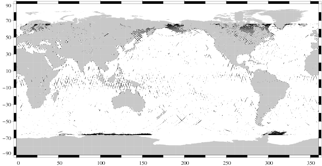
Valid data Jason-1 Cycle 302 (13/03/2010 / 23/03/2010)
