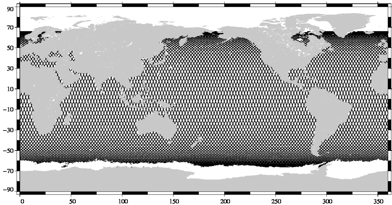
Valid data Jason-1 Cycle 351 (12/07/2011 / 22/07/2011)
